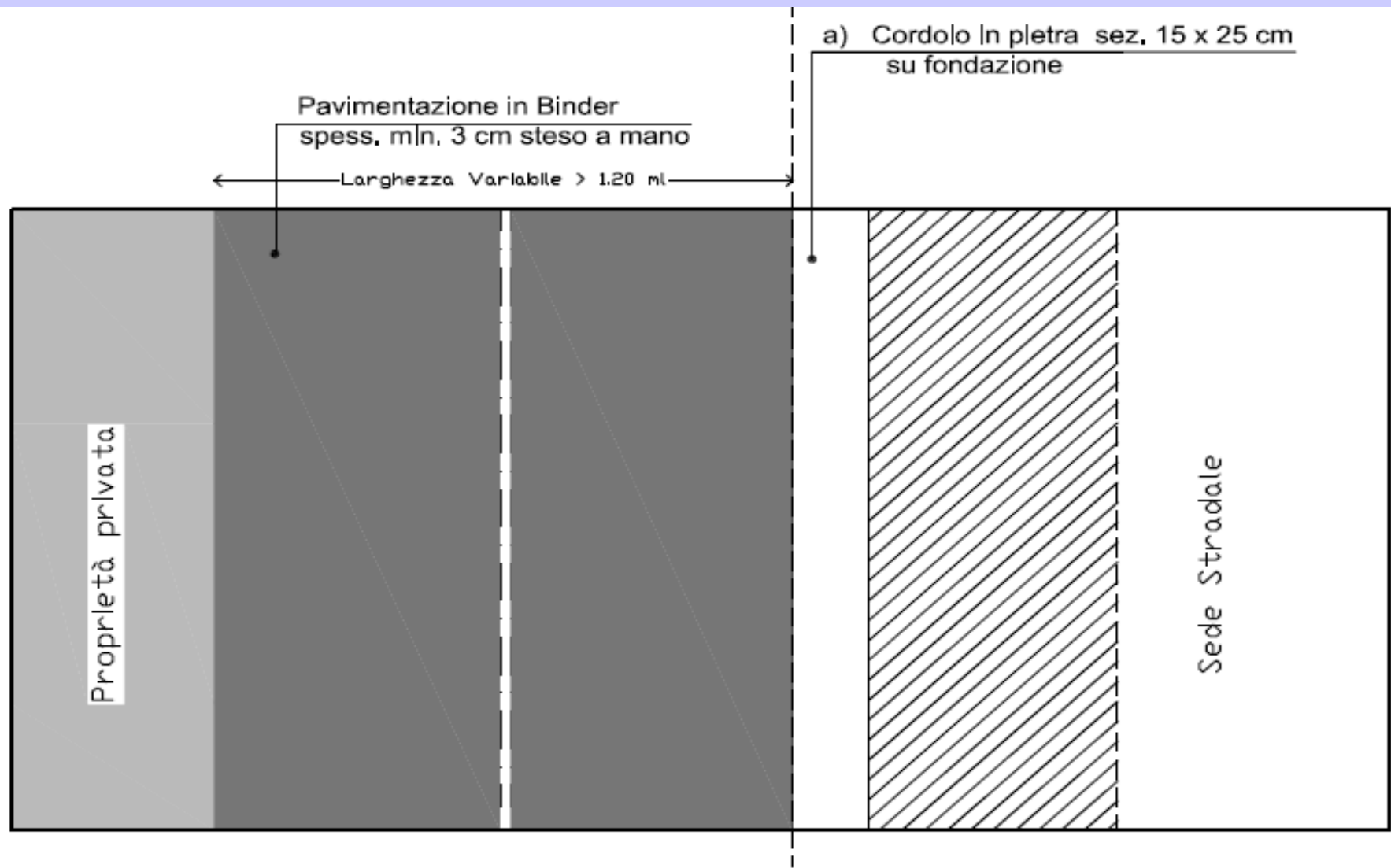
Pianta Particolare MarciapiEDE
